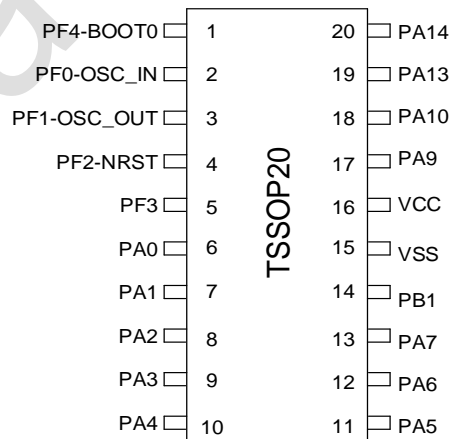
图 3-14 TSSOP20 Pinout3 PY32F030F3xPx
