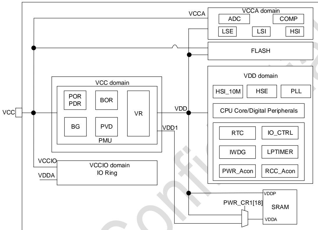
图 2-2 电源框图
