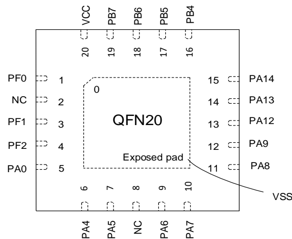
图 3-11 QFN20 Pinout3 PY32F030F3xUx
