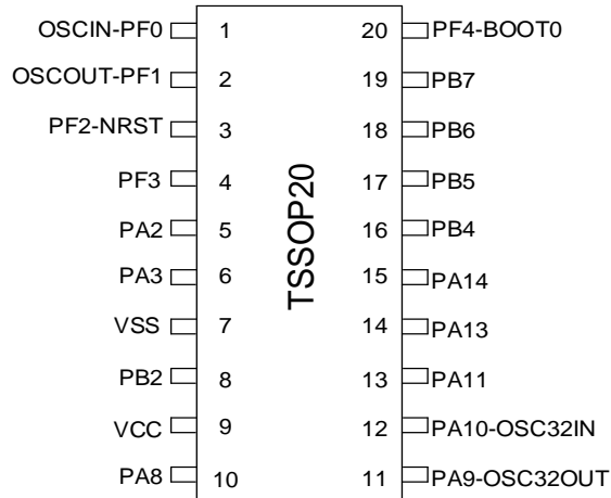
图 3-12 TSSOP20 Pinout1 PY32F030F1xPx
