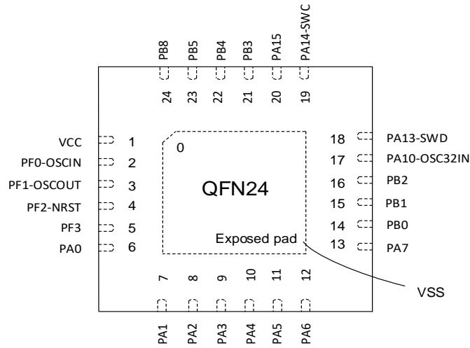
图 3-6 QFN24 Pinout1 PY32F030E1xUx-E
